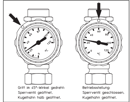
Abb. 30: Kugelhahn
