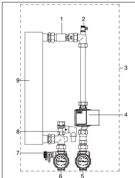
Abb. 9: Sekundärkreislauf
