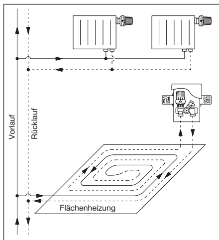
Abb. 6.2 Einbauposition
