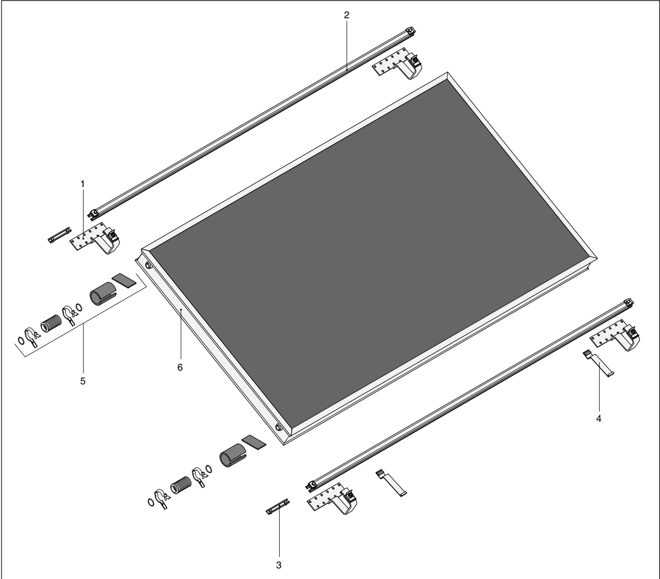
Abb. 12: Erweiterungsset Aufdachmontage
