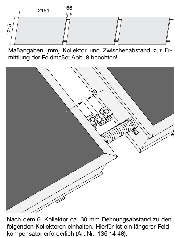
Abb. 8: Kollektorabstände
