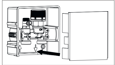
Abb. 8: Bauabdeckung aufsetzen
