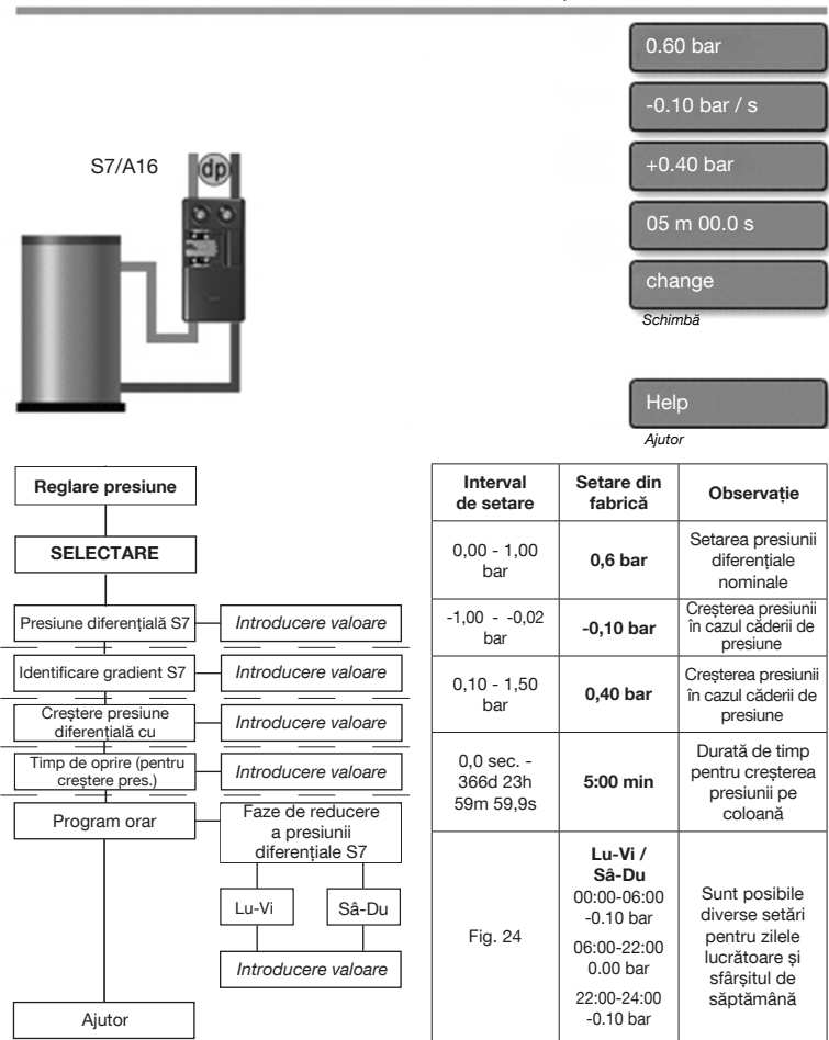
Reglarea presiunii diferențiale pe coloană Differential pressure control in the riser
