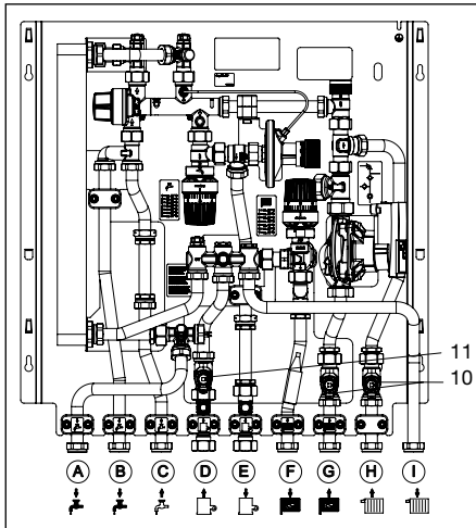
Abb. 8.1 Einbauposition Schmutzfänger
