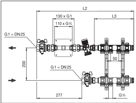
Abb. 3 Wärmemengenzähler-Anschluss-Set, Durchgangsform, und „Multidis SH“ Edelstahl-Verteiler für Heizkörperanbindung, Baulängen
