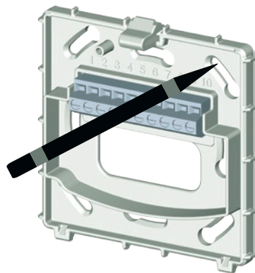
Abb. 8: Montageplatte montieren
