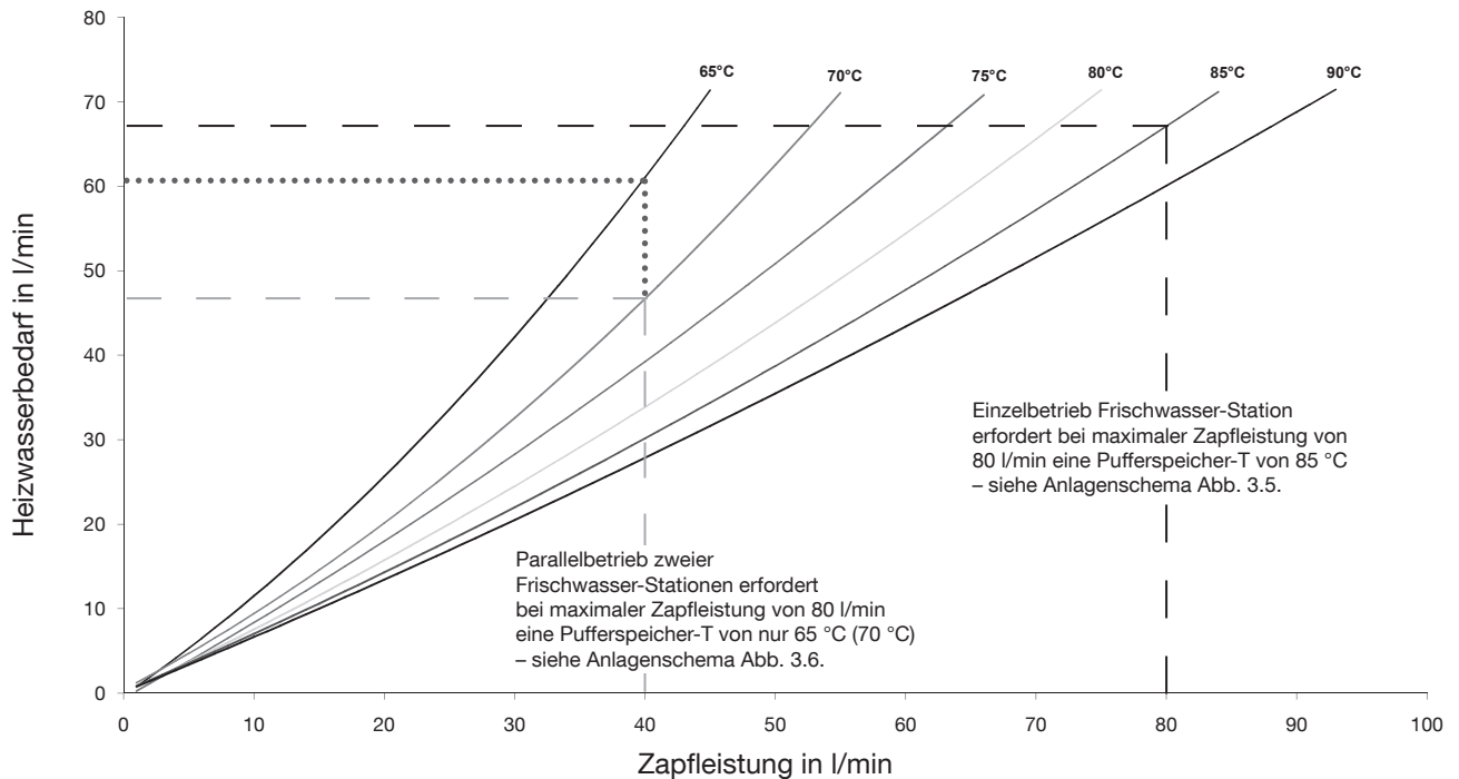
Abb. 3.4: Typischer Anwendungsfall „Trinkwassererwärmung 10 °C auf 60 °C“ (max. Zapfleistung von 80 l/min)*
