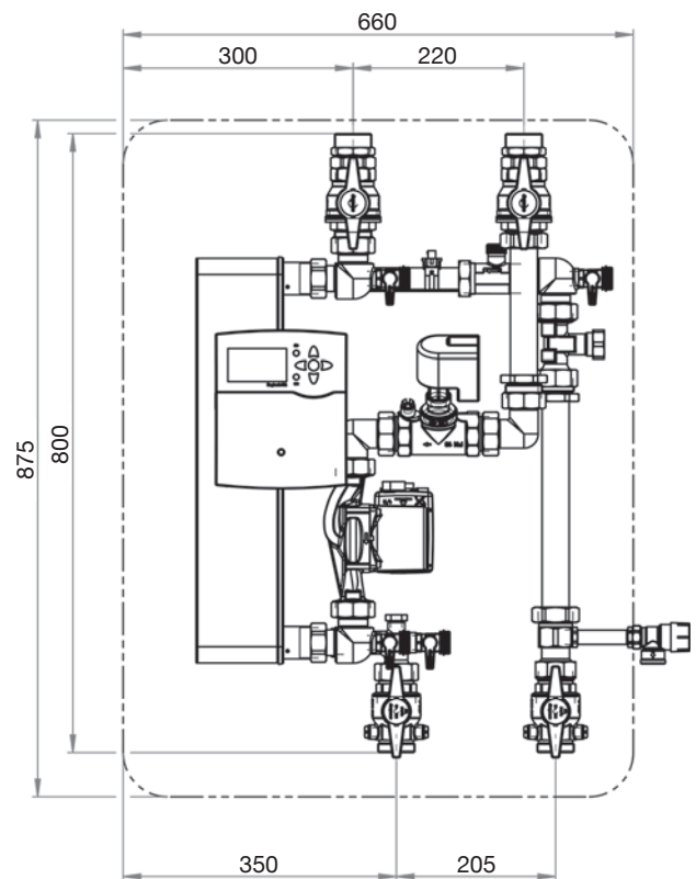
Abb. 3.8: Abmessungen „Regumaq X-80“ (Front)
