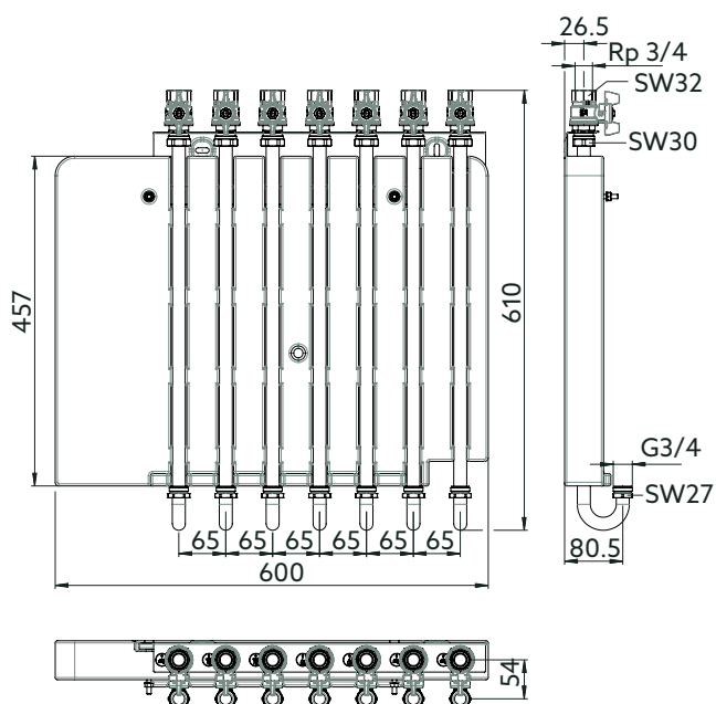
Fig. 2: Dimensions
