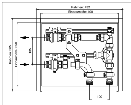
Abb. 3.1: Abmessungen seitliche Anbindung
