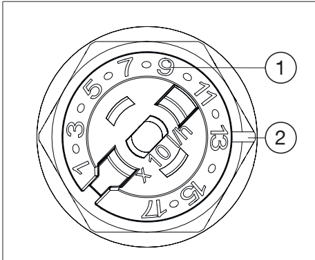
Abb. 7: Einstellung Ventileinsatz „QM“
