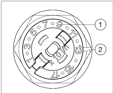
Fig. 7: Réglage du mécanisme « QM »
