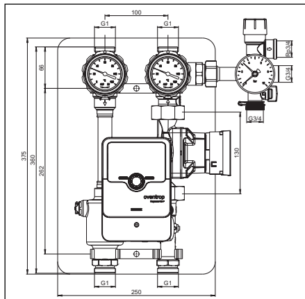
Abb. 4.4 Solarstation „Regusol ELH-130“ DN 25
