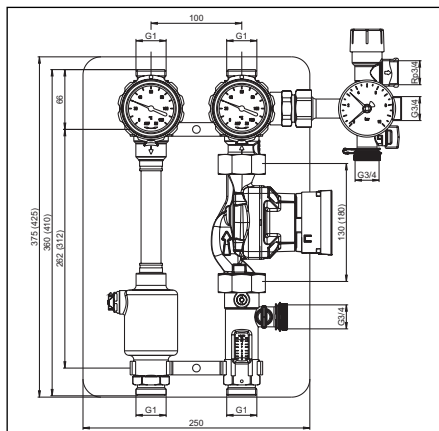
Abb. 4.3 Solarstation „Regusol LH-130 (180)“ DN 25
