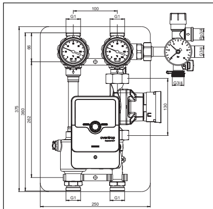
Fig. 4.4 Station solaire «Regusol ELH-130» DN 25
