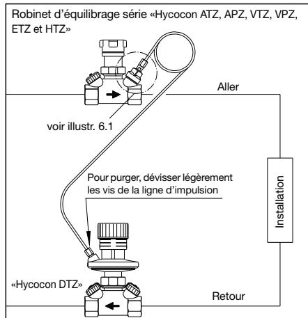
Illustr. 6.2: «Hycoco DTZ» Montage sur le retour
