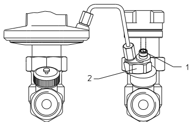
Illustr. 6.1: «Hycoco DTZ» Illustration du raccordement de la ligne d'impulsion, montage sur le retour
