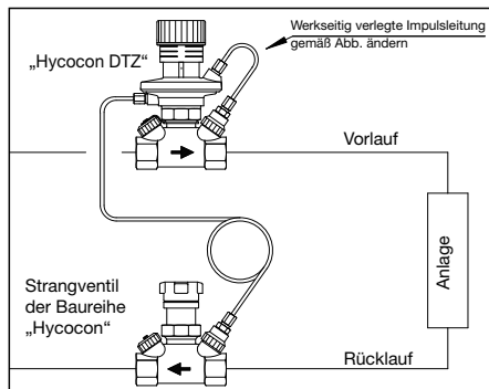
Abb. 6.3: „Hycoccon DTZ“. Einbau im Vorlauf (nur DN 32 + DN 40)
