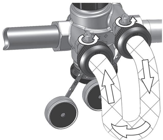
Fig. 10 - Svutamento, riempimento, risciacquo e sfiato della sezione dell'impianto completa
