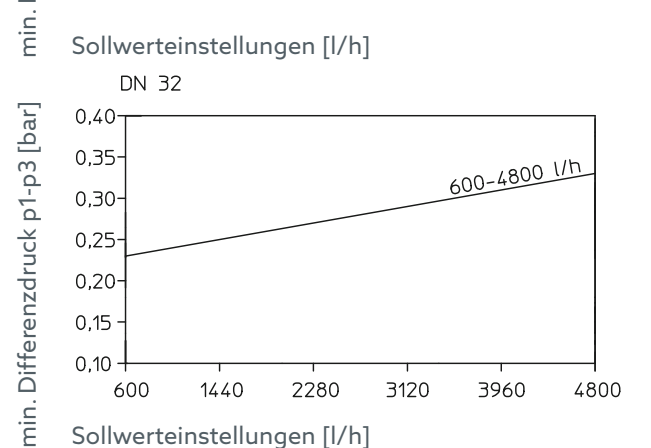
Abb. 13: Mindest-Differenzdrücke
