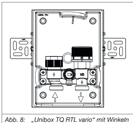
Abb. 8: „Unibox TQ RTL vario“ mit Winkeln
