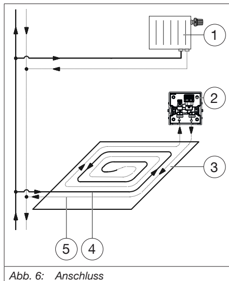
Abb. 6: Anschluss
