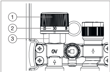
Abb. 4: Handrad
