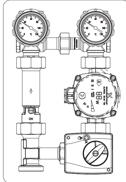
Regumat M3-130
